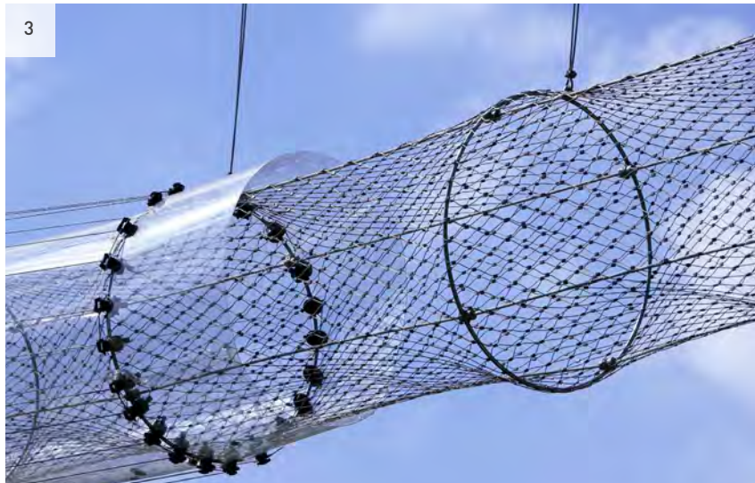
Bewegungsfreiheit von A nach B mit Tunnelnetzen Freedom of movement from A to B with tunnel mesh
