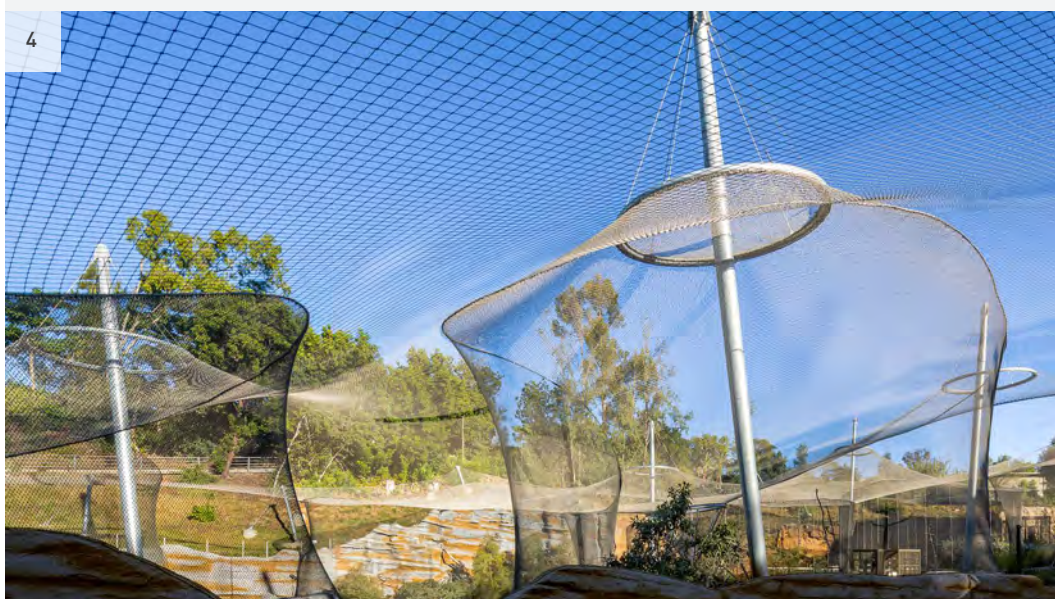
Wandnetze mit optimiertem, und somit optisch reduziertem Dachnetzanschluss Wall mesh with optimized and thus almost imperceptible attachment to the roof mesh
