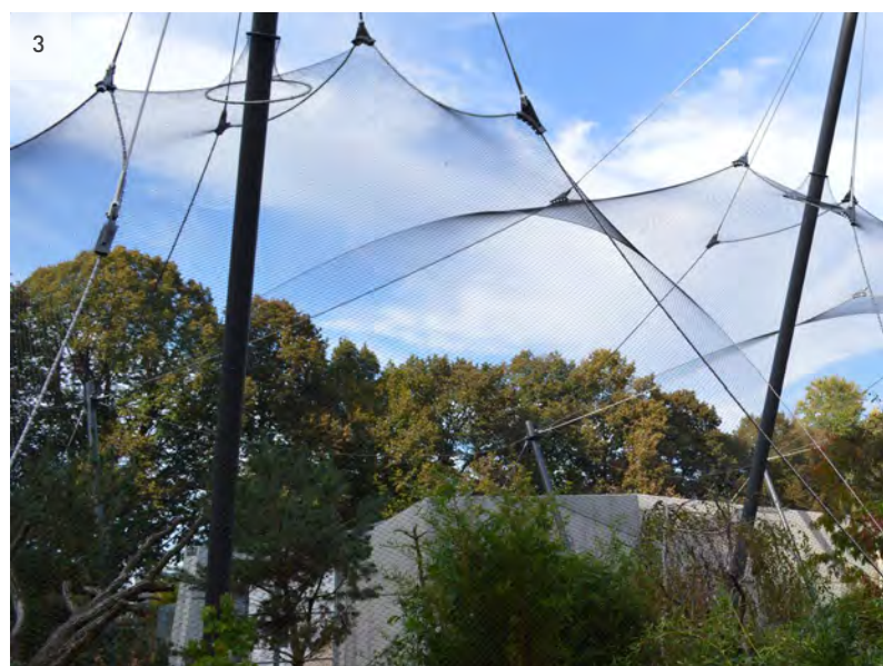
Begehbare Voliere für Watvögel mit außenliegender Zugseil-Konstruktion
